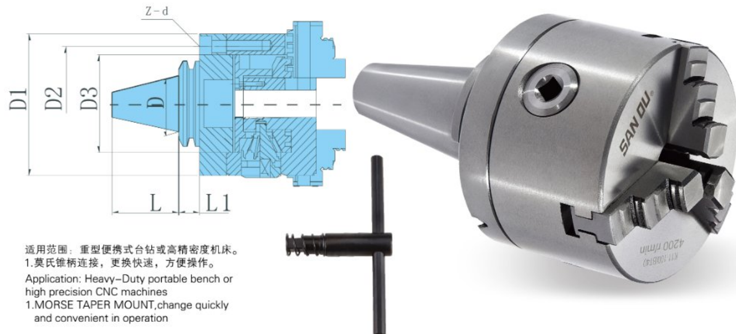
尺寸、性能参数 Dimension characteristic parameters
