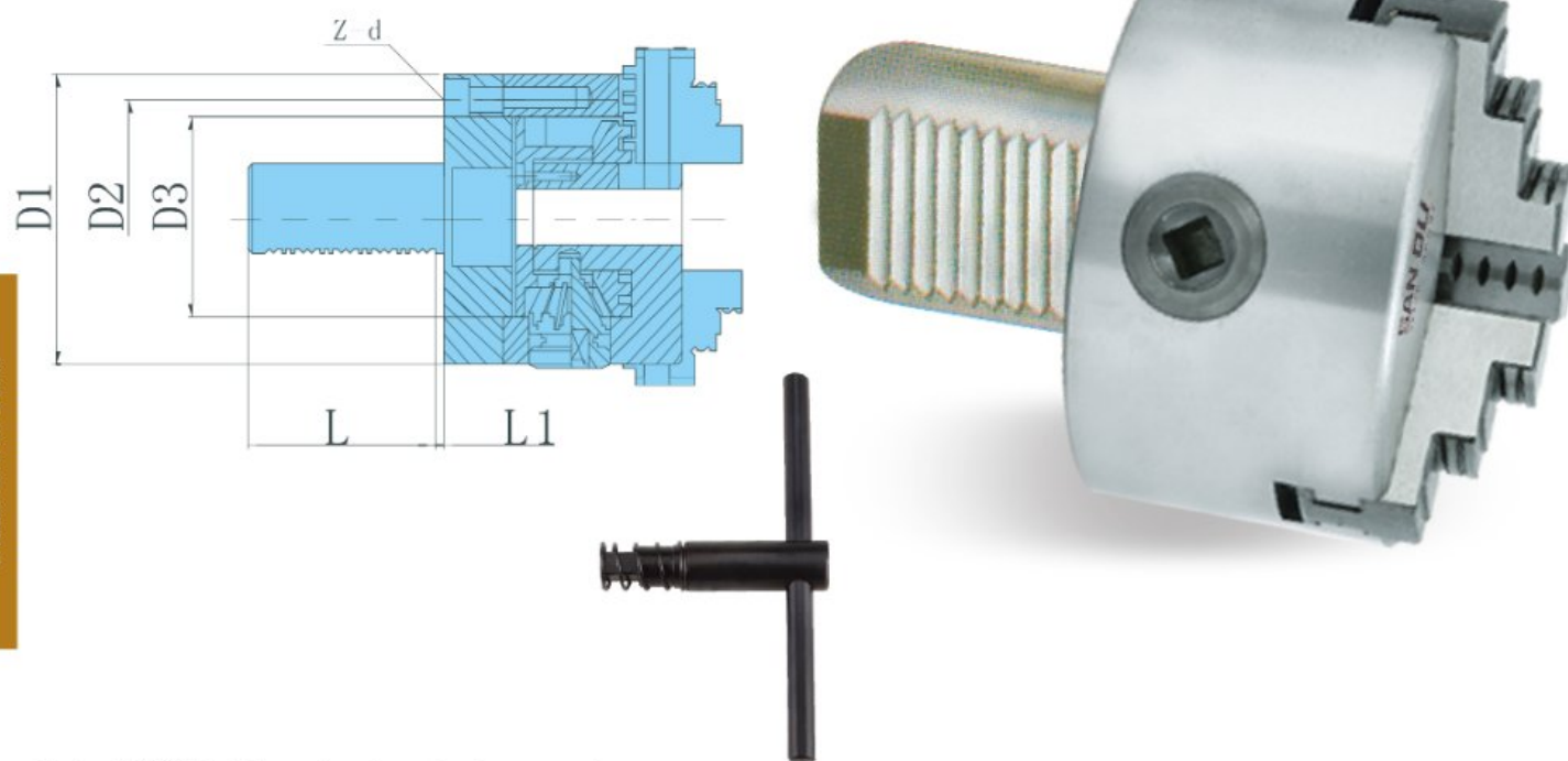
尺寸、性能参数 Dimension characteristic parameters
