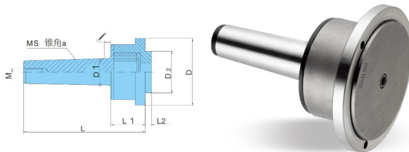
尺寸、性能参数 Dimension characteristic parameters
