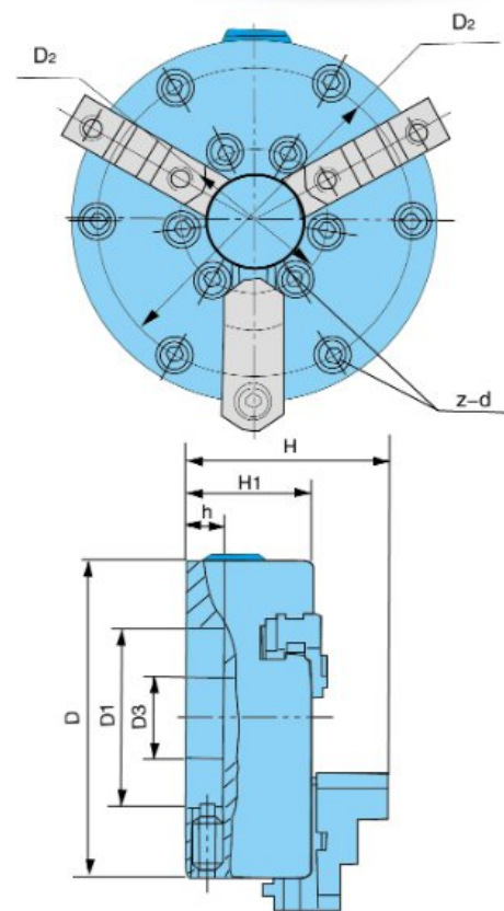
尺寸、性能参数 Dimension characteristic parameters
